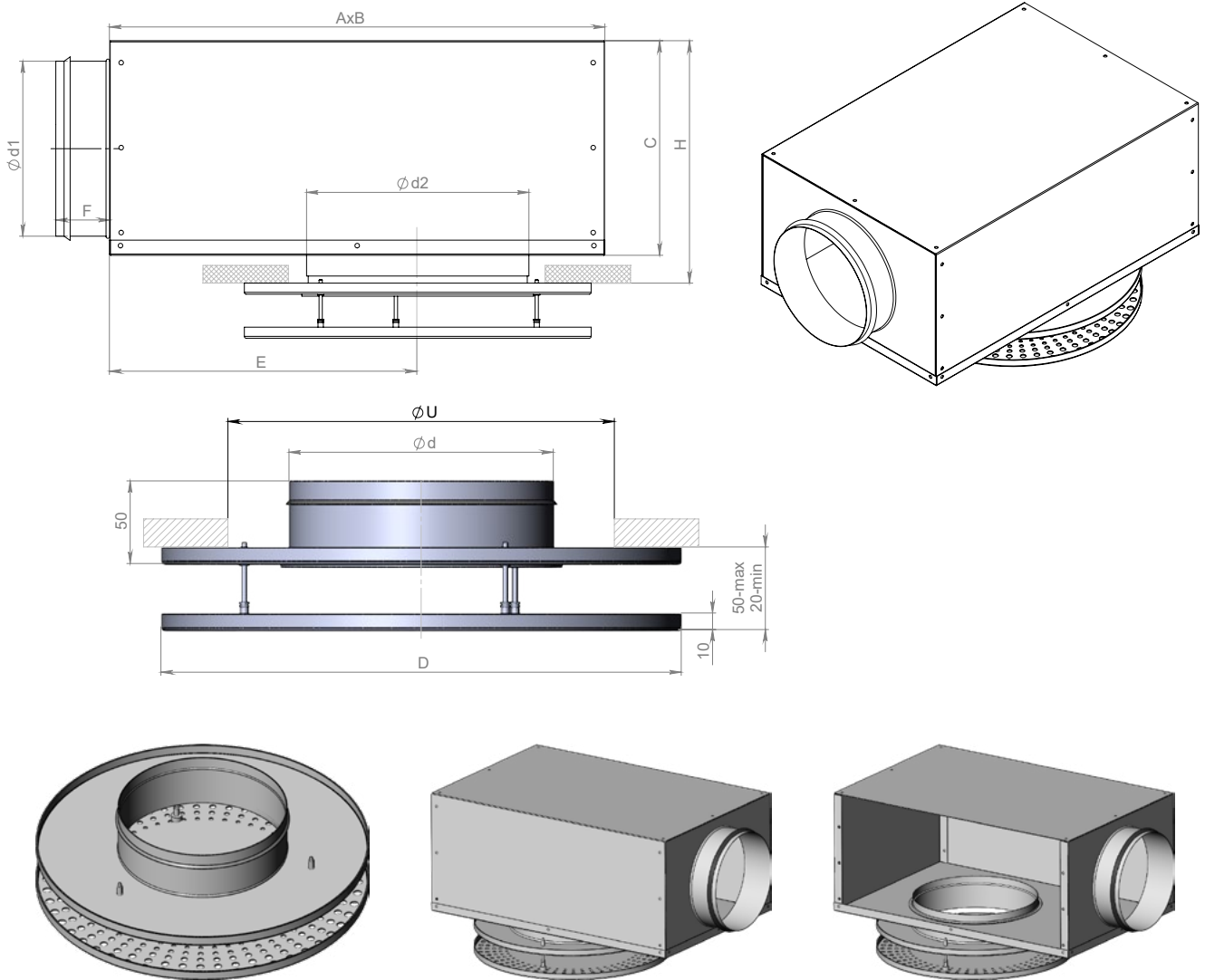
Габаритно-посадочные размеры диффузора TSK
